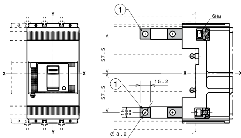
КРЕПЛЕНИЕ НА 50 мм
