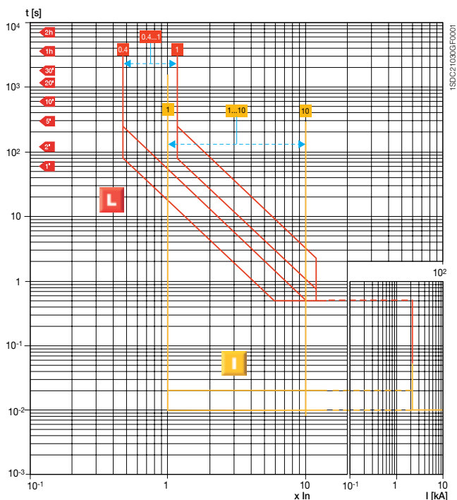
ХТ4 Еkip N-LS/I Функции L-I
