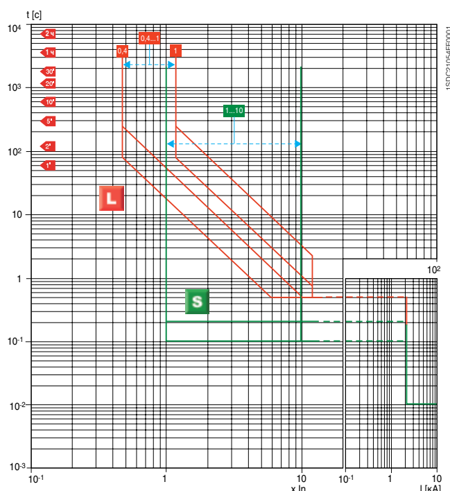
ХТ4 Еkip N-LS/I Функции L-S
