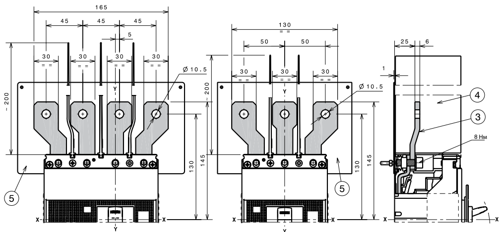
3 ПОЛЮСА
