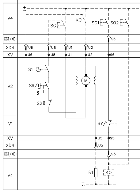
Привод MOD
