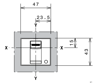
A=79 3-4 ПОЛЮСА
