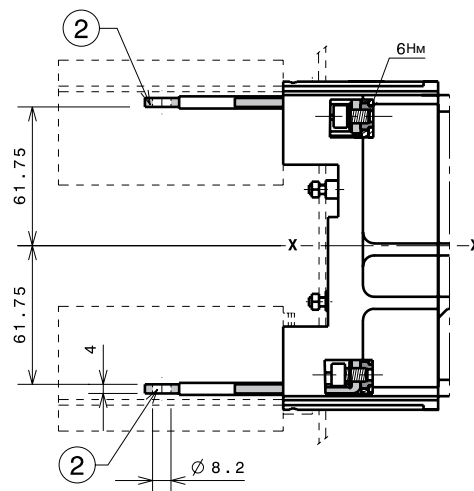
КРЕПЛЕНИЕ НА 50 мм
