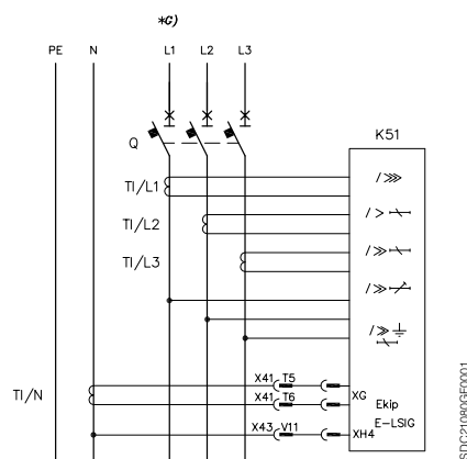
Трехполюсный стационарный автоматический выключатель XT4 с расцепителем защиты Ekip E-LSIG и внешним датчиком тока в нейтрали
