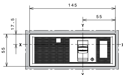
B=124 C=144 4 ПОЛЮСА
