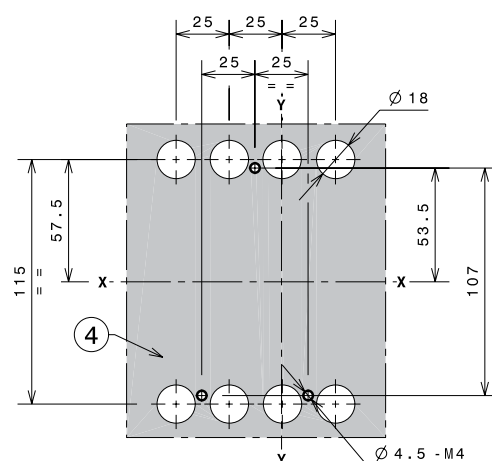
4 ПОЛЮСА
