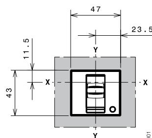
A=79 3-4 ПОЛЮСА
