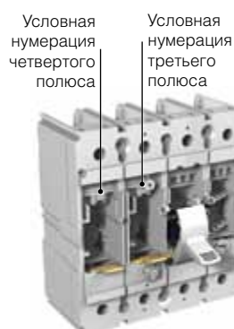
Четырехполюсный выключатель
