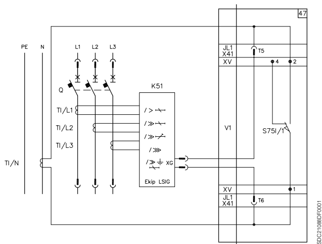
Схема, рекомендуемая для трехполюсного выкатного или выкатного автоматического выключателя с трансформатором тока на нейтральном проводнике вне автоматического выключателя
