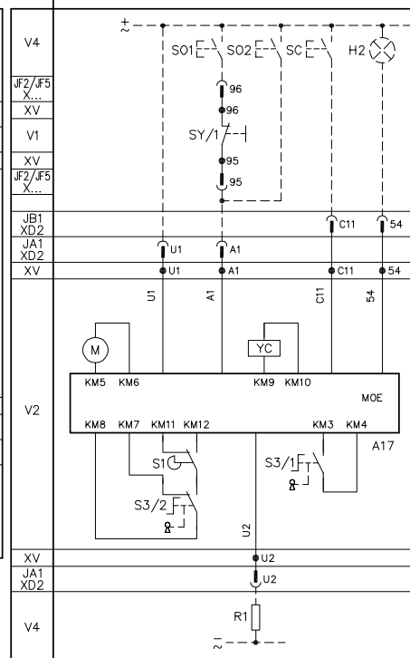
Привод МОЕ или МОЕ-Е *H)
