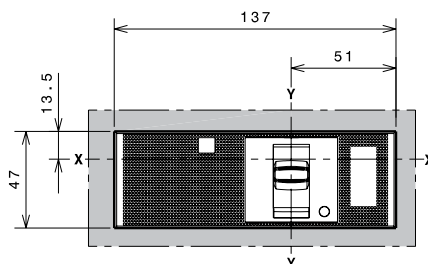
B=121 C=141 4 ПОЛЮСА
