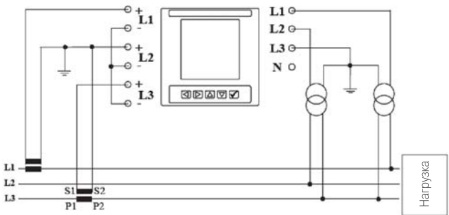
Ввод с 2 трансформаторами тока и 2 трансформаторами напряжения (Агон)
