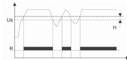
Диаграмма работы E 236-US 1.1 и US 2.1
