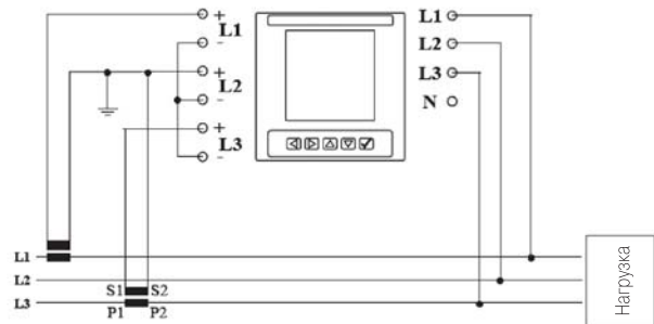
Ввод с 2 трансформаторами тока
