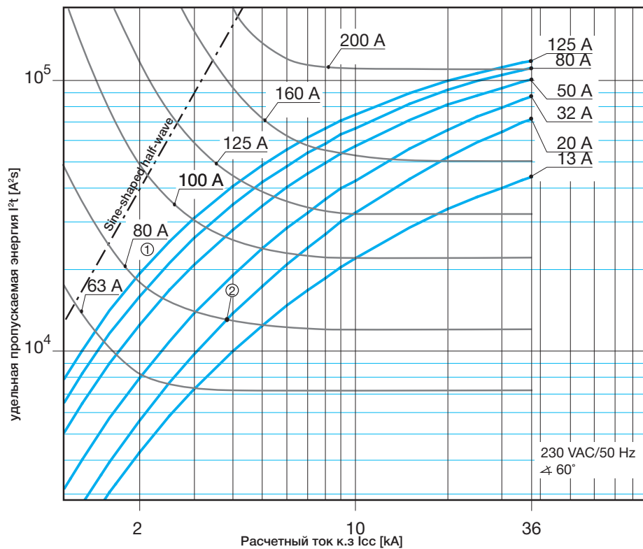
S800 N характеристики В, С и D 230 В удельная пропускаемая энергия
