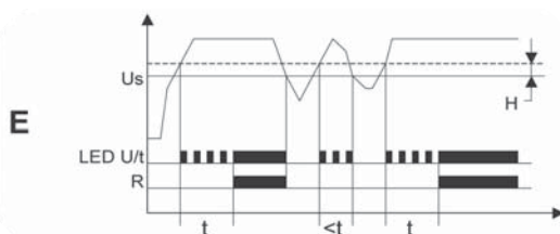
Диаграмма работы E 236-US 1.1D
