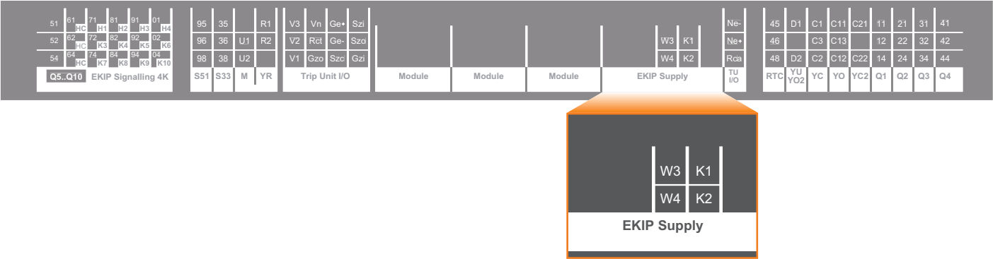
31) Клеммы для подключения внешнего источника питания 24 В пост. тока и локальная шина
