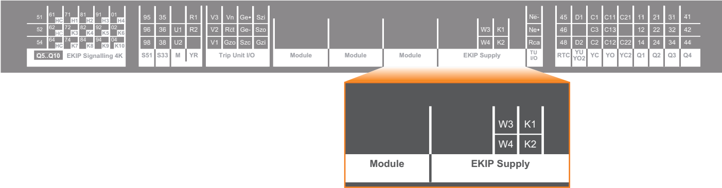
33) Модуль вентиляции Ekip Fan 24 В пост. тока
