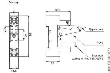
CR-PSS — винтовое соединение
