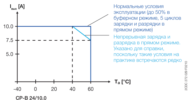
Зависимость номинального тока от температуры
