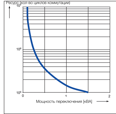
CR-M с 4 переключающими контактами
