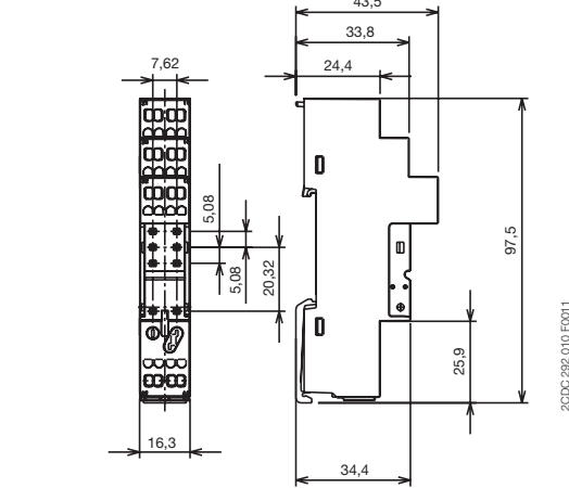
CR-PLC — винтовое соединение
