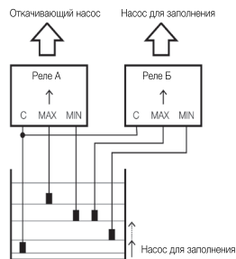
Наполнение с помощью резервного насоса
