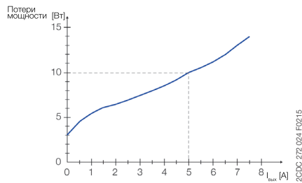
Усредненная зависимость потерь мощности от выходного тока
