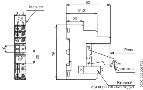
CR-PLS — винтовое соединение
