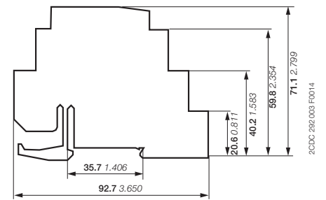
Разделитель для CR-S
