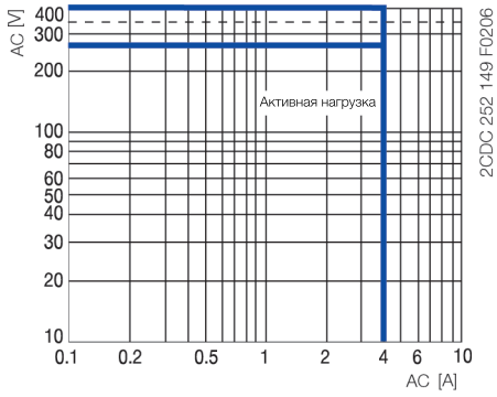
Нагрузка AC (резистивная)
