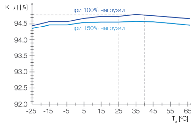
Усредненная зависимость КПД от температуры окружающего воздуха
