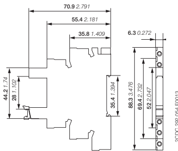
Цоколь с винтовыми клеммами для интерфейсных реле серии CR-S
