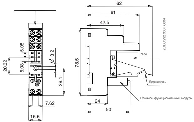
CR-PLSx — винтовое соединение
