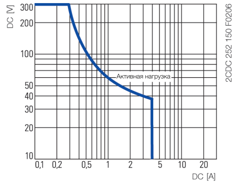
Нагрузка DC (резистивная)
