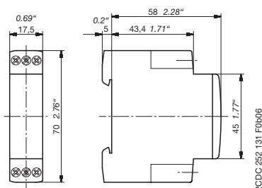
Устройства СТ-D с 1 ПК или с 2 н. о. контактами
