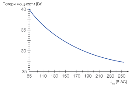
Усредненная зависимость потерь мощности от входного напряжения AC
