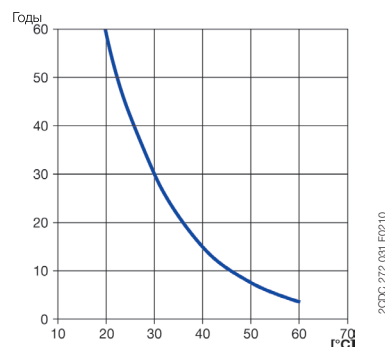
Срок службы конденсатора в зависимости от температуры
