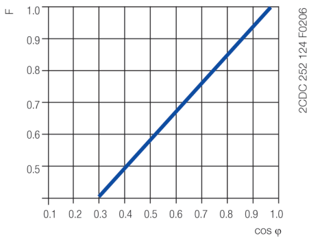
Коэффициент пересчета F при индуктивной нагрузке AC
