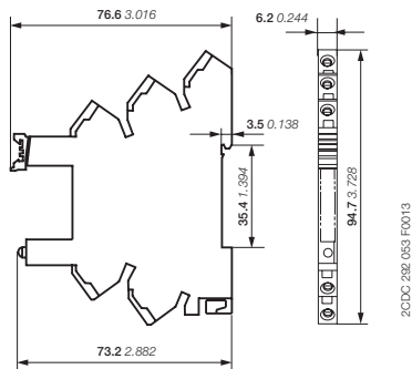
Цоколь с пружинными клеммами для интерфейсных реле серии CR-S
