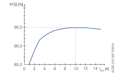
Усредненная зависимость КПД от выходного тока
