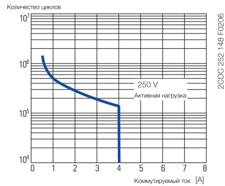
Срок службы контактов
