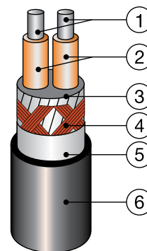
Конструкция нагревательного кабеля
