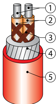
Конструкция нагревательного кабеля
