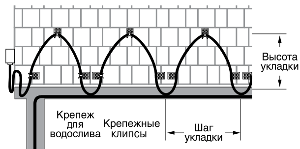
Вид сбоку на крышу с установленной системой антиобледенения.
