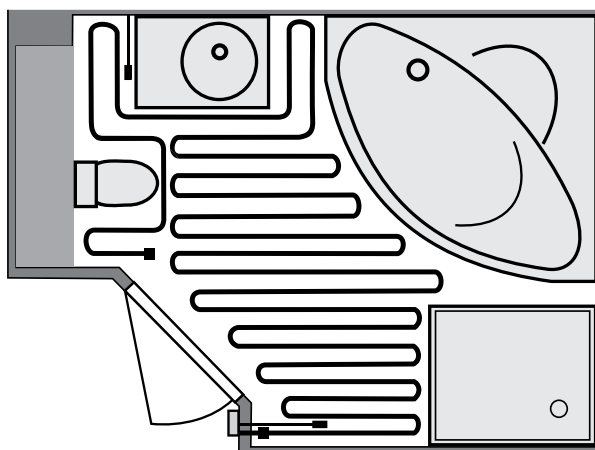
Рис.унок 3. Схема укладки нагревательного кабеля
