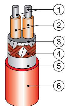
Конструкция нагревательного кабеля
