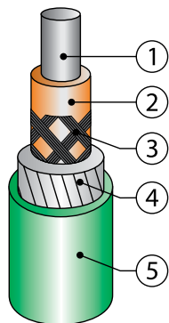
Конструкция нагревательного провода
