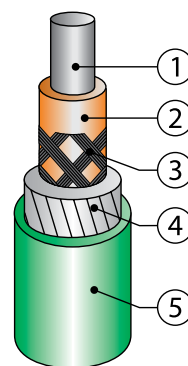
Конструкция нагревательного провода
