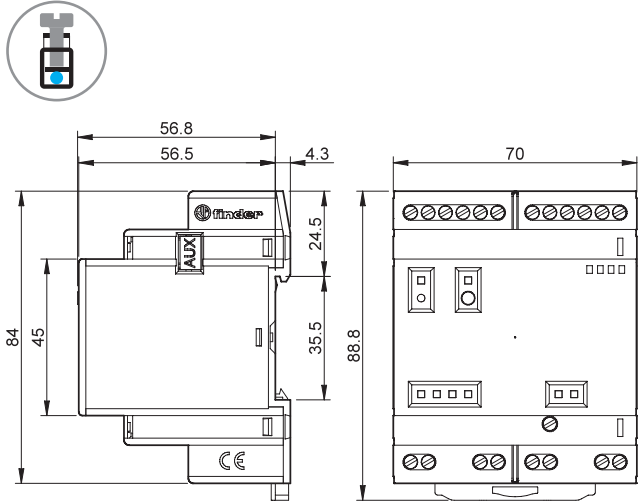
Тип 8А.04-8300 Винтовые клеммы
