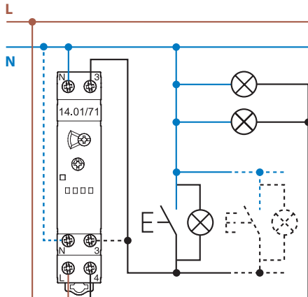
3-проводное соединение
