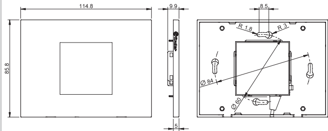
Монтаж в 3-модульные настенные коробки
