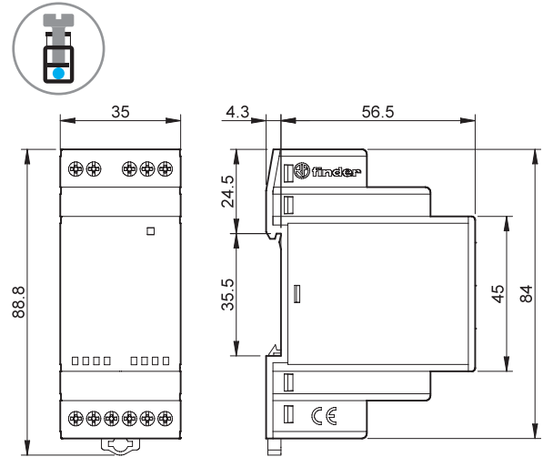
Тип 70.51.0.240.N032 Винтовые клеммы
