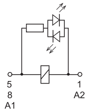
C: Опция 74 СИД (неполяризованный DC)
