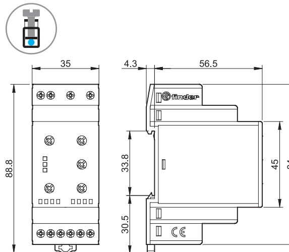
Тип 70.42 Винтовые клеммы
