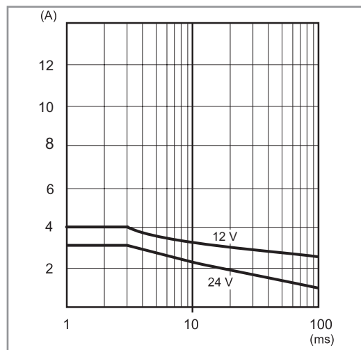
P78-3 Зависимость пикового тока на выходе от времени (78.36) - 12 В
