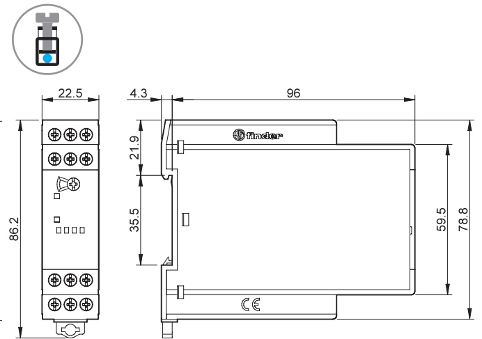
Тип 70.92 Винтовые клеммы
