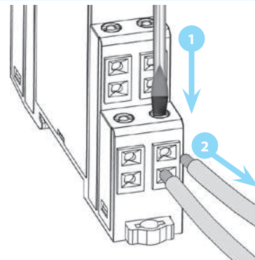
Отключение электрического провода
