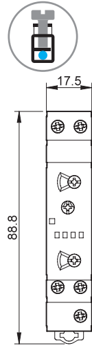
Тип 80.82 Винтовые клеммы
