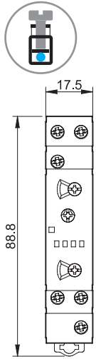
Тип 80.01/80.51 Винтовые клеммы
