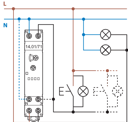
4-проводное соединение
