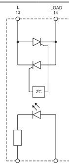
Упрощенная принципиальная схема
