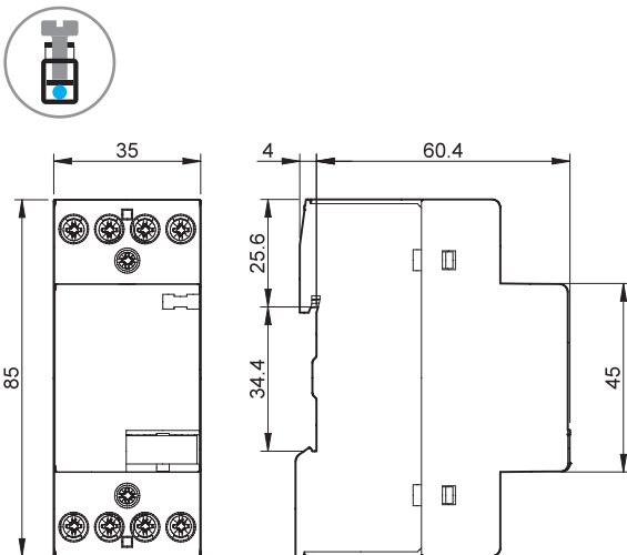
Тип 22.74 Винтовые клеммы
