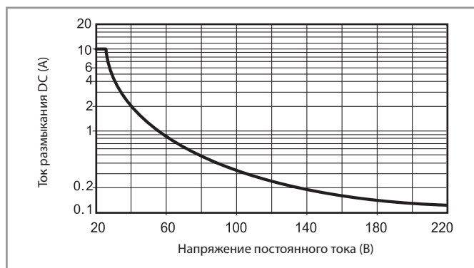
H 8А - Макс. отключающая способность DC1
