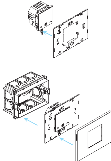
Монтаж в 3-модульные настенные коробки
