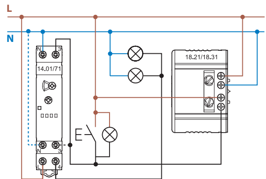
4-проводное соединение (только с 18.21.8.230.0300 или 18.31.8.230.0300)
