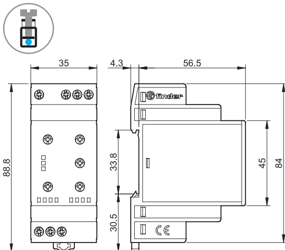
Тип 70.41 Винтовые клеммы
