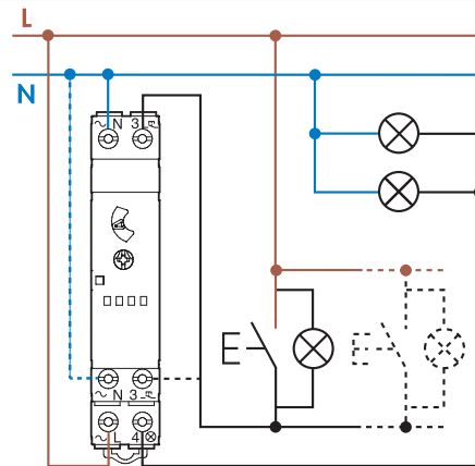
4-проводное соединение
