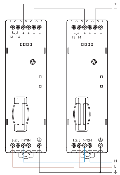
Последовательное подключение
