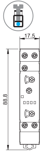
Тип 80.71 Винтовые клеммы
