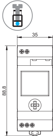
Тип 12.51/12.81 Винтовые клеммы
