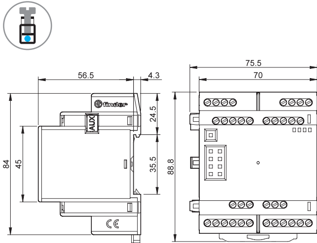
Тип 8А.58-1600 Винтовые клеммы
