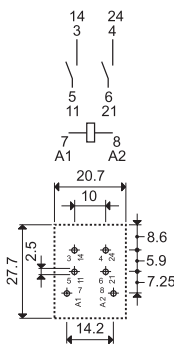
56.42-0300 Вид со стороны выводов
