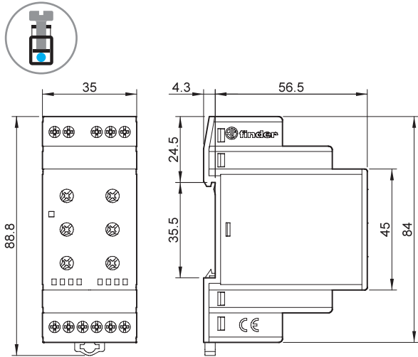
Тип 70.51.0.240.2032 Винтовые клеммы
