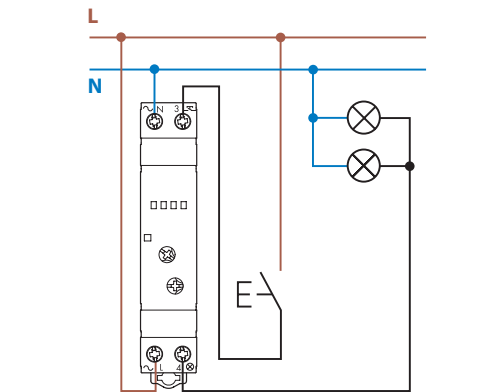
Тип 15.81 - 4-проводное соединение
