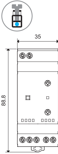
Тип 11.41 Винтовые клеммы
