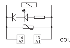
Пример: АС
