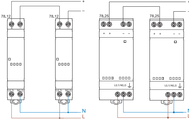
последовательное соединение
