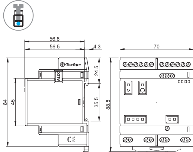
Тип 8А.04-8310/8320 Винтовые клеммы
