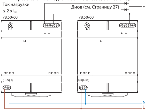
Параллельное подключение (78.50/60 только)
