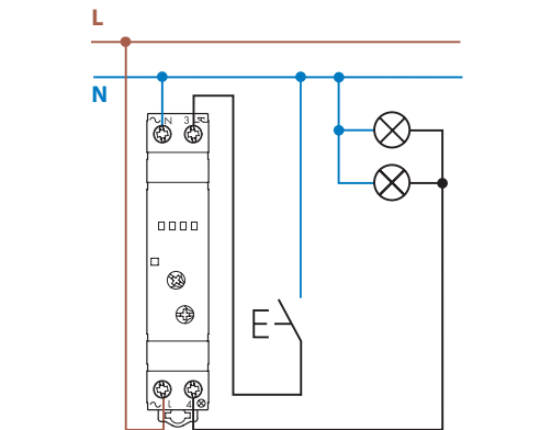
Тип 15.81 - 3-проводное соединение
