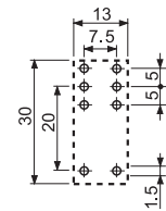
95.15.2 Вид сбоку
