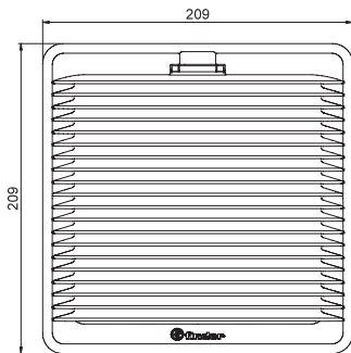
Тип 7F.xx.x.xxx.4250 Клеммы Push-in
