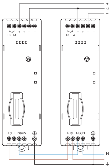
Сдвоенное подключение
