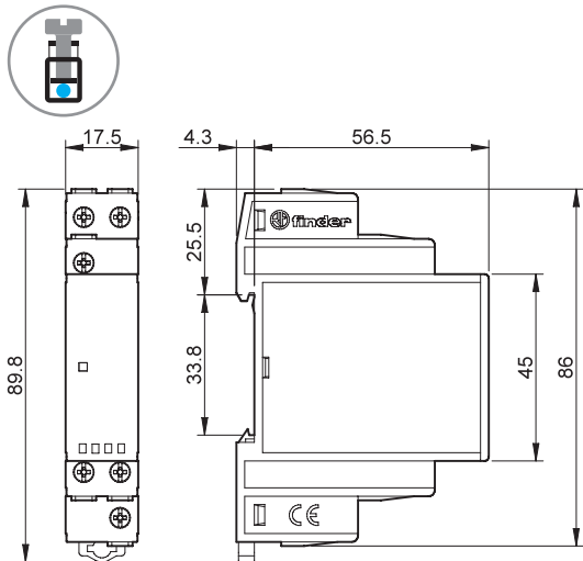
Тип 70.61 Винтовые клеммы
