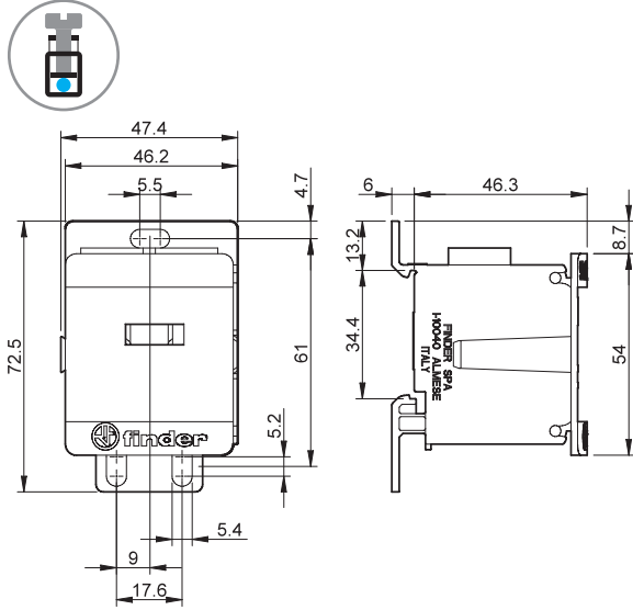
Тип 9D.01.5.175.0210 Винтовые клеммы
