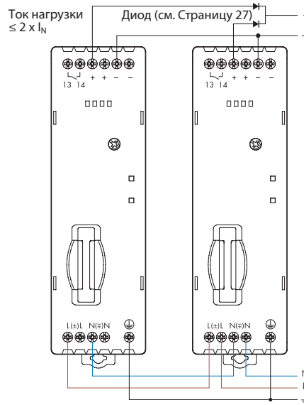
Параллельное подключение
