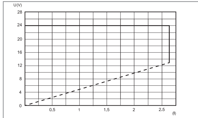
FB78-2 Зависимость выходного напряжения от выходного тока (78.60)
