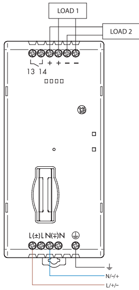
Типовое подключение
