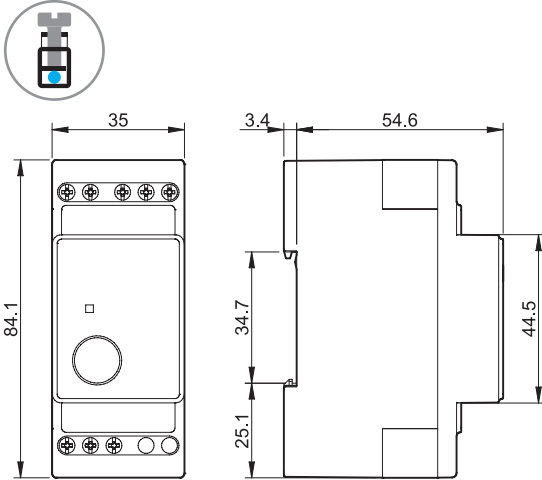
Тип 13.11 Винтовые клеммы
