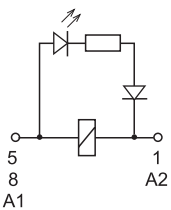
C: Опция 54 светодиод (AC)
