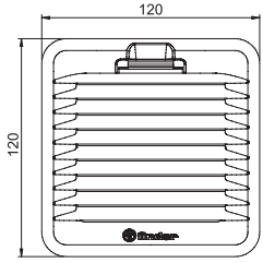
Тип 7F.xx.x.xxx.2055 Клеммы Push-in
