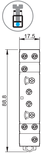
Тип 80.91 Винтовые клеммы
