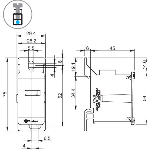
Тип 9D.01.5.250.0111 Винтовые клеммы
