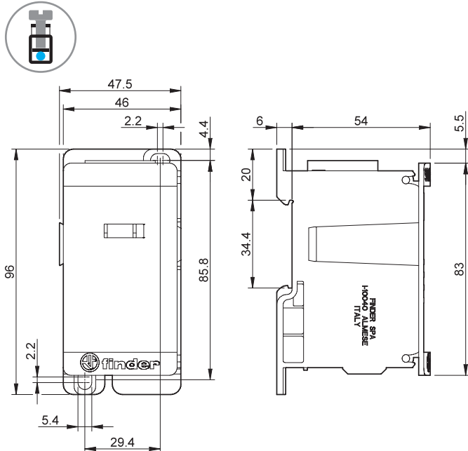
Тип 9D.01.5.400.0111 Винтовые клеммы
