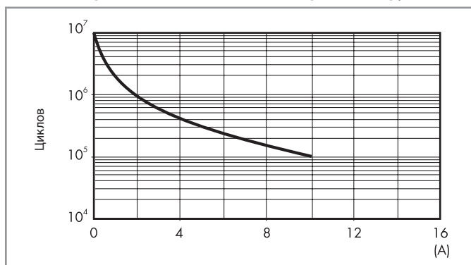
F 8А - Электрическая долговечность (АС) при ном. нагрузке
