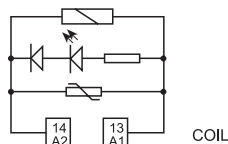
Пример: AC
