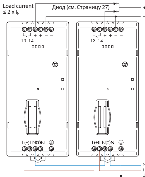
Параллельное подключение
