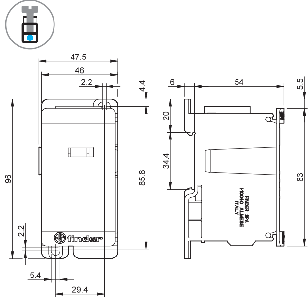
Тип 9D.01.5.250.0111 Винтовые клеммы
