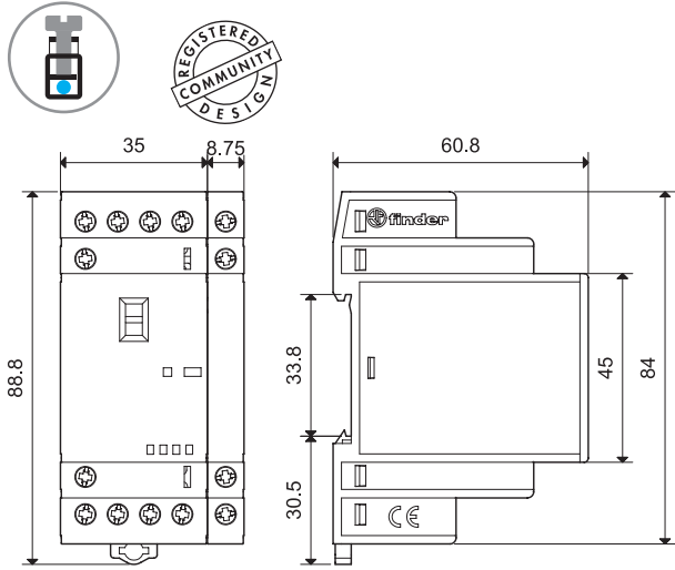
Тип 22.34 + 022.33/022.35 Винтовые клеммы
