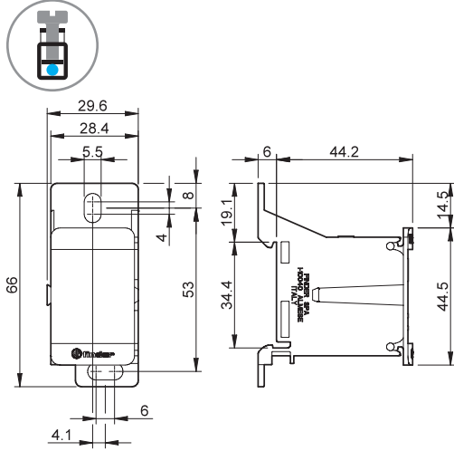
Тип 9D.01.5.080.0304 Винтовые клеммы
