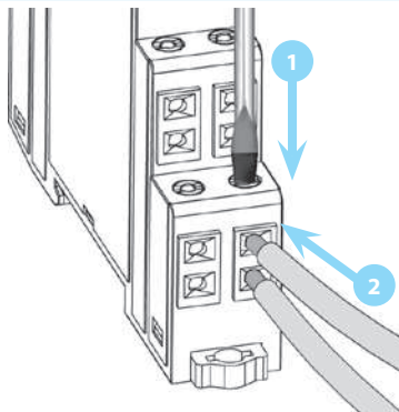
Подключение с многожильным проводом (без отвертки в случае одножильного провода)
