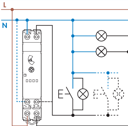
3-проводное соединение
