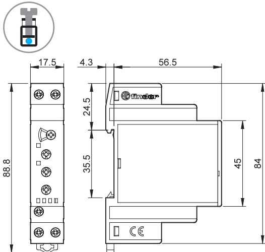
Тип 70.41 Винтовые клеммы
