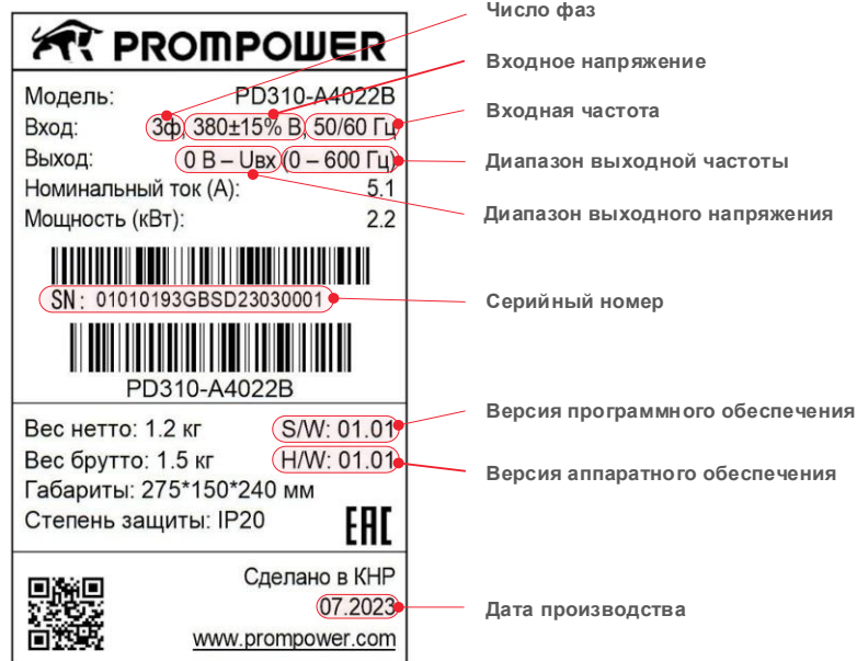
Рисунок 2-2 Описание шильдика
