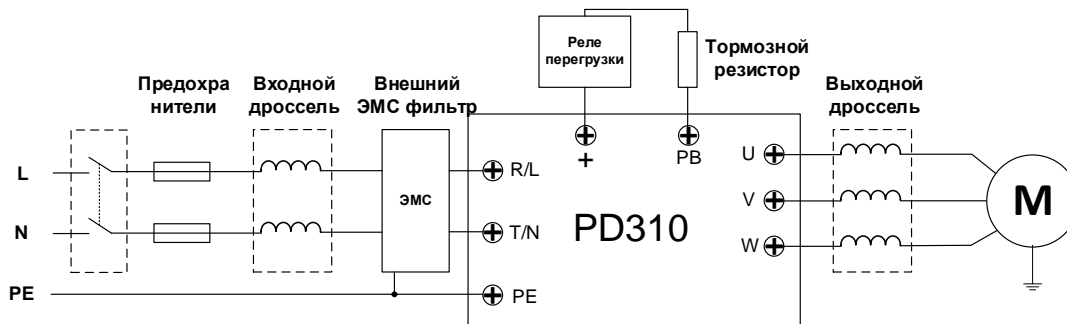
Рисунок 4-17 Схема подключения однофазных моделей АВ
