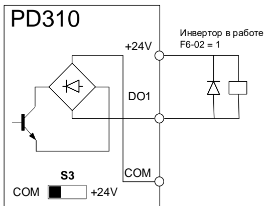
Рисунок 4-31 Схема подключения дискретного выхода с использованием внутреннего питания преобразователя в режиме NPN
