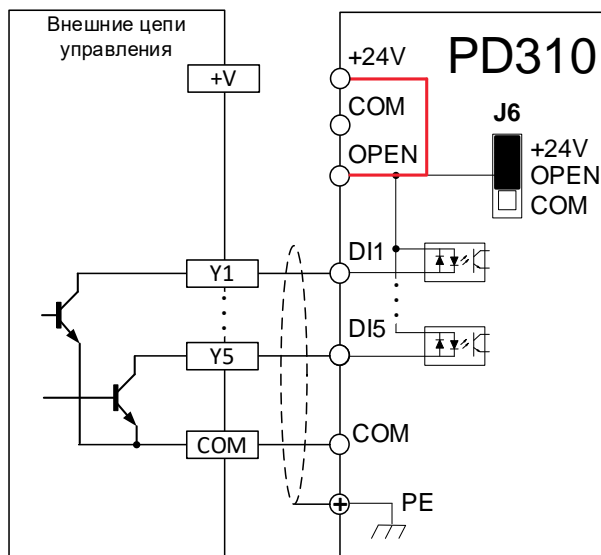
Рисунок 4-26 Режим NPN, использование внутреннего источника питания
