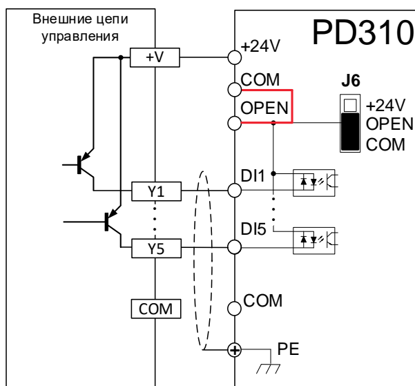
Рисунок 4-27 Режим PNP, использование внутреннего источника питания
