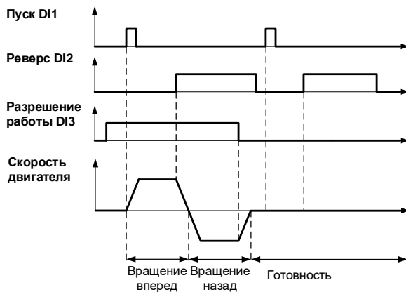
Рисунок 9-43 Формирование команд управления с дискретных входов
