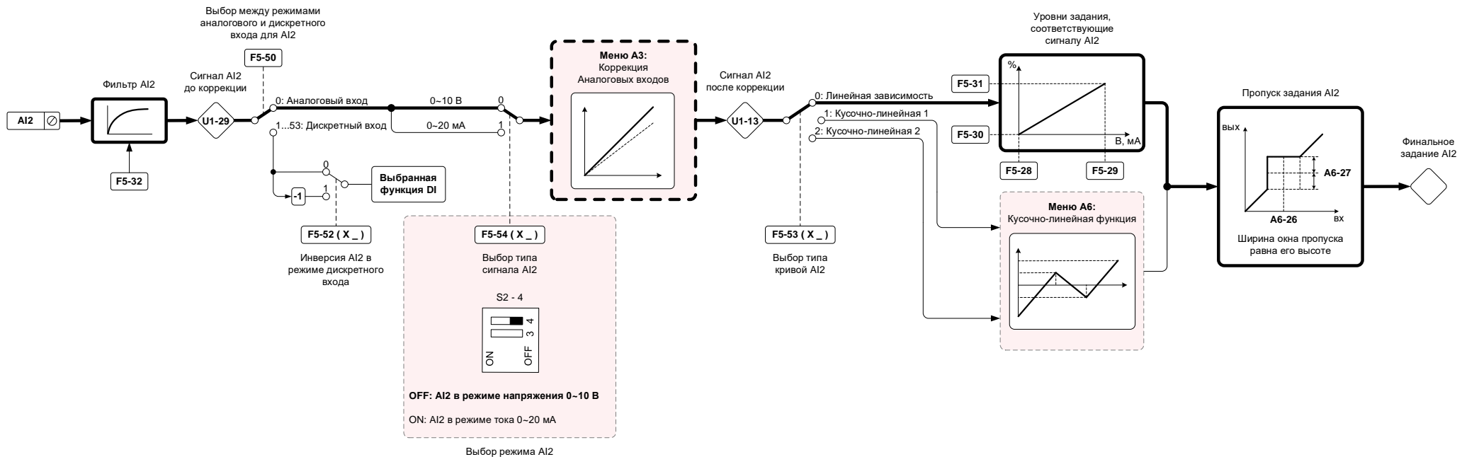
Рисунок 9-16 Функциональные схемы аналоговых входов
