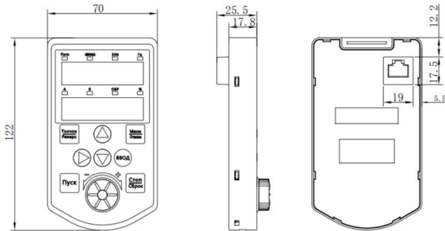
Рисунок 3-13 Габаритные размеры внешней панели управления
