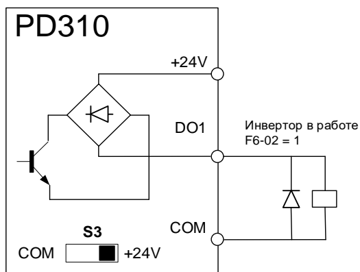
Рисунок 4-32 Схема подключения дискретного выхода с использованием внутреннего питания преобразователя в режиме PNP
