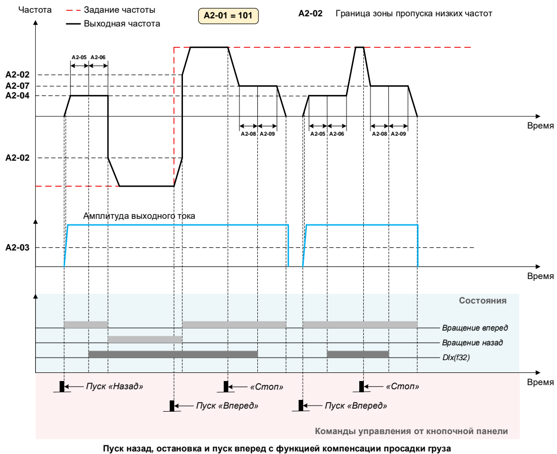
Рисунок 9-57 Временные диаграммы при использовании функции управления механическим тормозом с компенсацией просадки груза и пропуском низких частот
