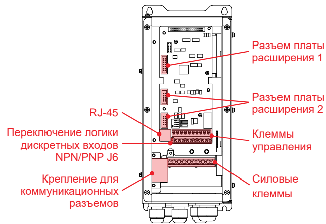
Рисунок 4-13 Расположение клемм преобразователей частоты IP54 PD310-D4007B, PD310-D4015B, PD310-D4022B, PD310-D4040B, PD310-D4055B
