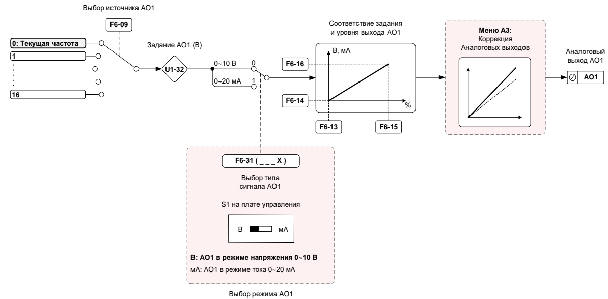
Оptionальная плата входов/выходов PD310IO1
