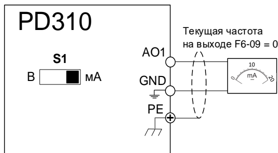
Рисунок 4-37 Схема подключения аналогового выхода в режиме 0~20 мА
