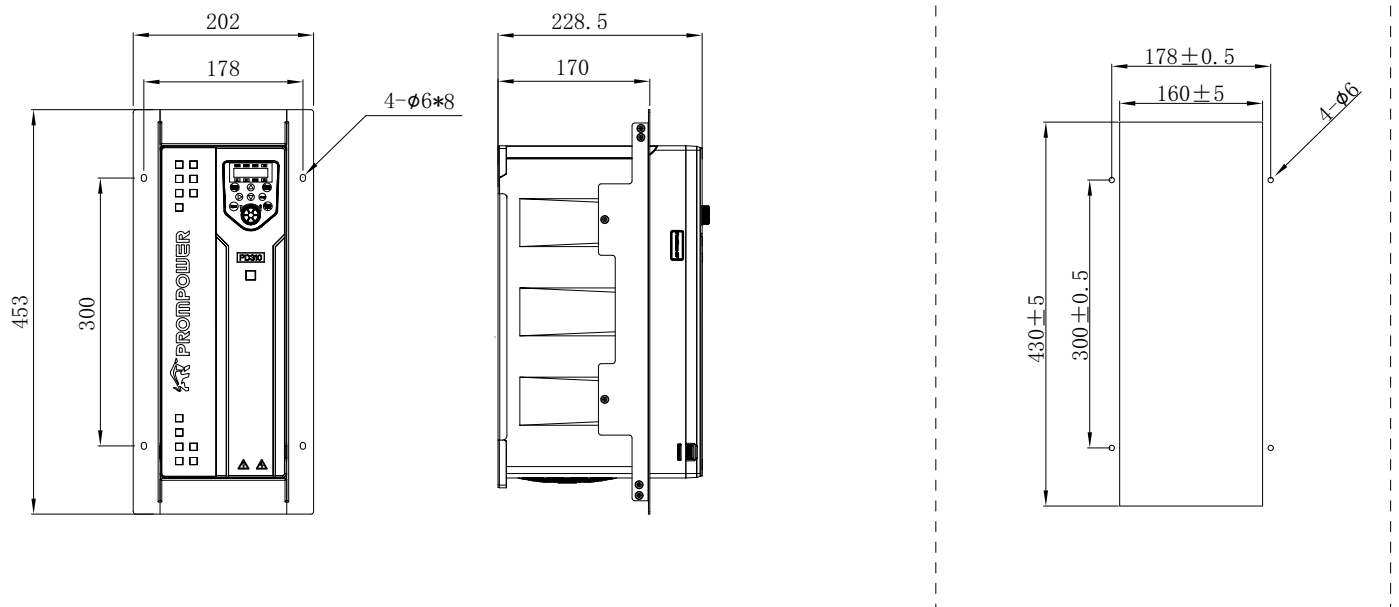
Рисунок 3-9 Монтажные размеры для установки в проем монтажной панели моделей 15-22 кВт
