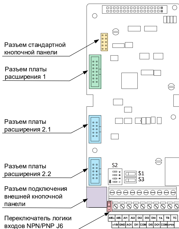
Рисунок 4-25 Расположение клемм управления и DIP-переключателя J6
