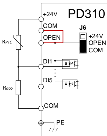
Рисунок 4-30 Подключение PTC датчика в режиме PNP
