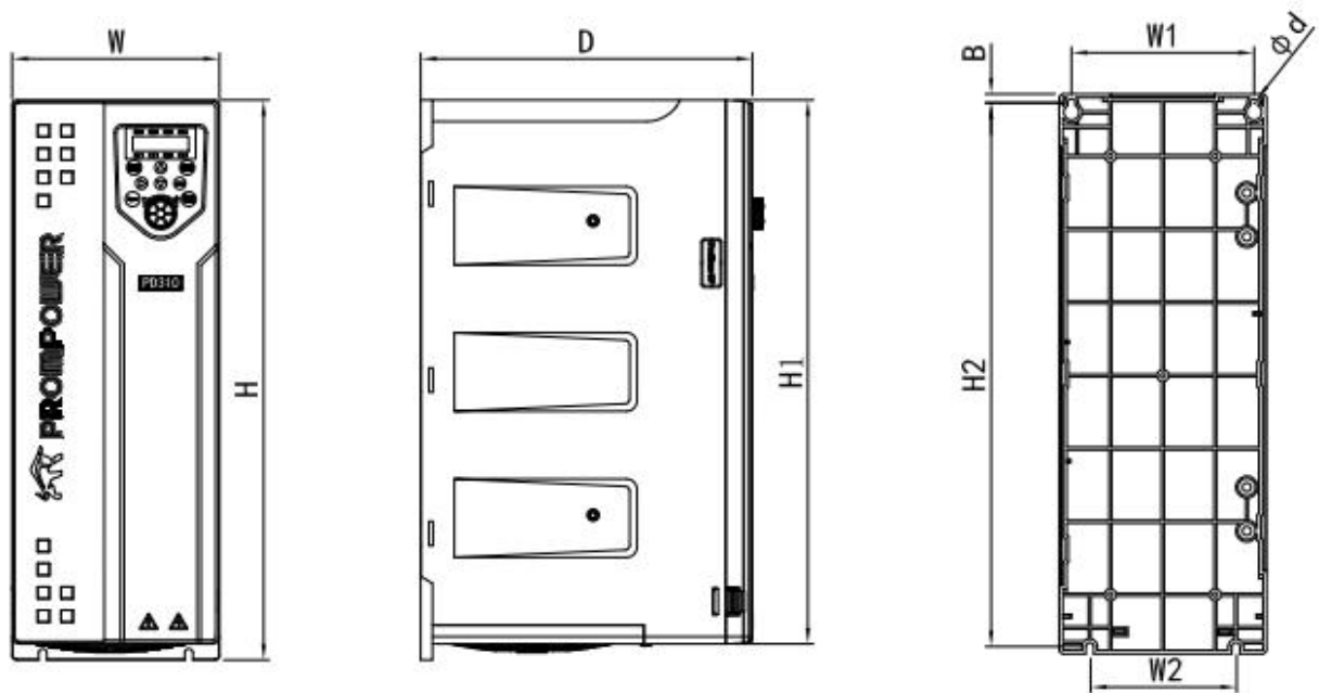
Рисунок 3-2 Габаритные размеры
