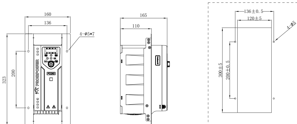
Рисунок 3-6 Монтажные размеры для установки в проем монтажной панели моделей 0,75-4 кВт
