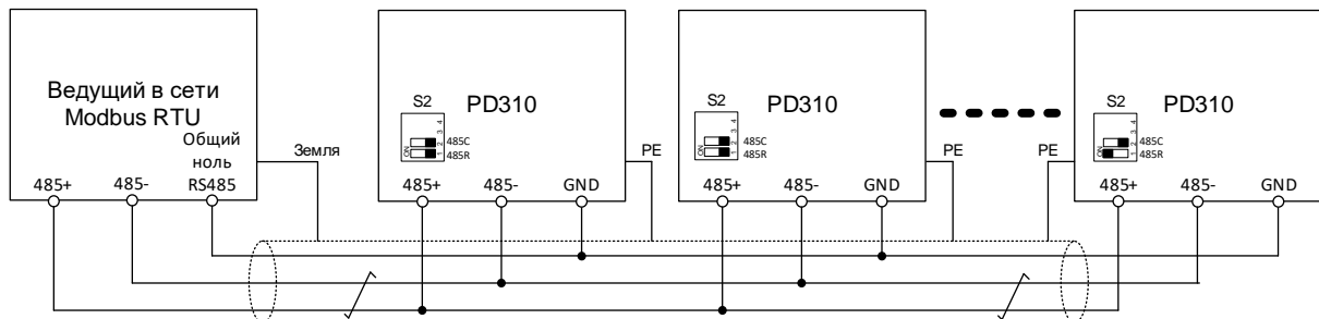
Рисунок 10-3 Подключение нескольких ПЧ в общую сеть RS-485
