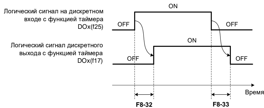
Рисунок 9-39 Временные диаграммы работы функции таймера
