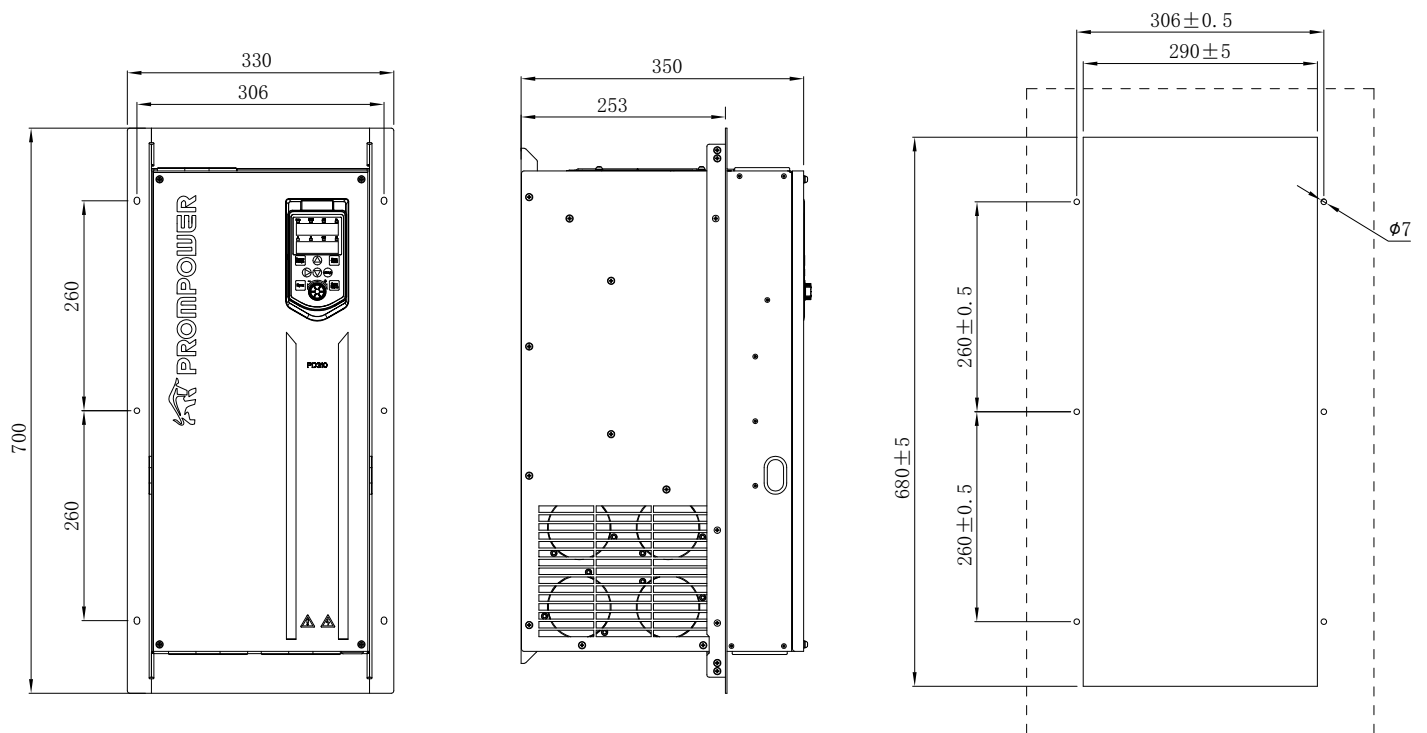
Рисунок 3-12 Монтажные размеры для установки в проем монтажной панели моделей 90-110 кВт
