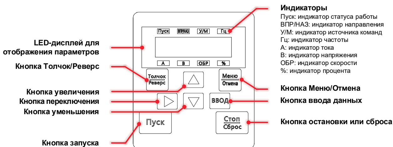
Рисунок 5-3 Однострочная кнопочная панель управления для ПЧ IP54
