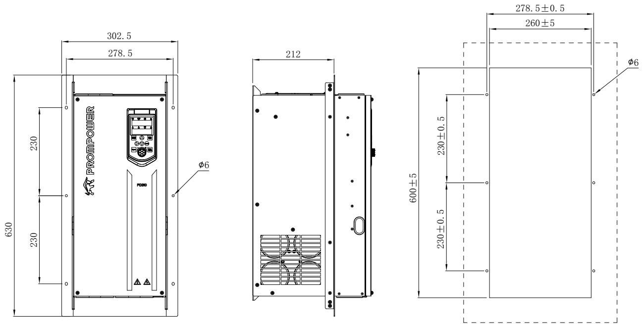
Рисунок 3-11 Монтажные размеры для установки в проем монтажной панели моделей 45-75 кВт
