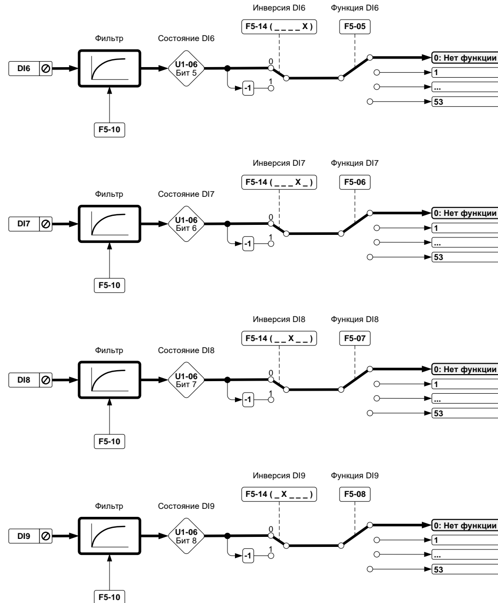
Рисунок 9-18 Функциональные схемы дискретных входов плат расширения (опционных)
