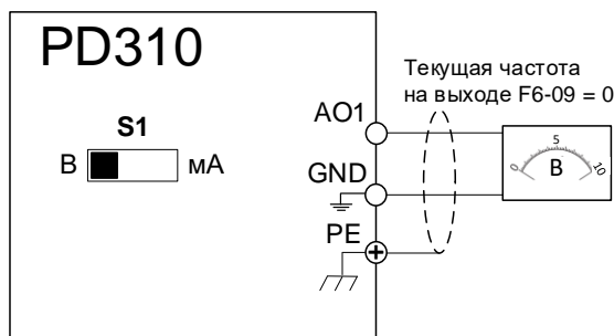
Рисунок 4-36 Схема подключения аналогового выхода в режиме 0~10 В
