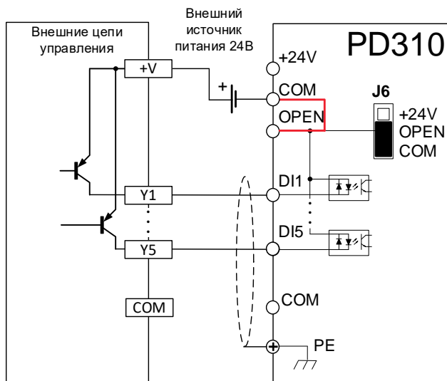
Рисунок 4-29 Режим PNP, использование внешнего источника питания
