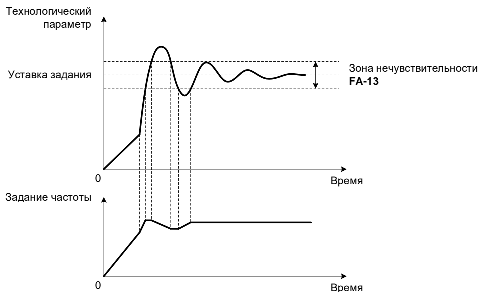
Рисунок 9-49 Работа ПИД-регулятора прямого действия с зоной нечувствительности
