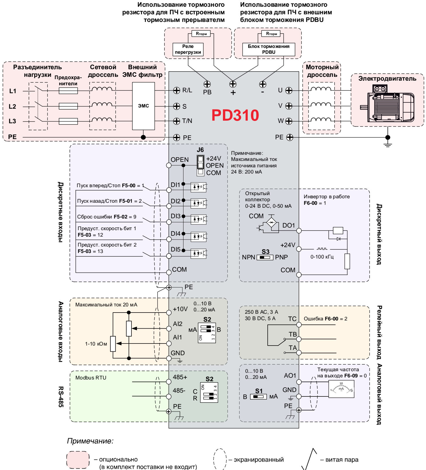
Рисунок 4-24 Типовая схема электрических подключений
