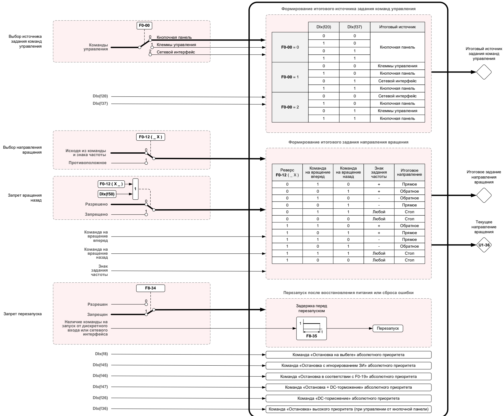
Рисунок 9-4 Контроллер управления
