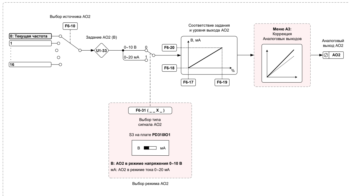
Рисунок 9-30 Функциональные схемы аналоговых выходов
