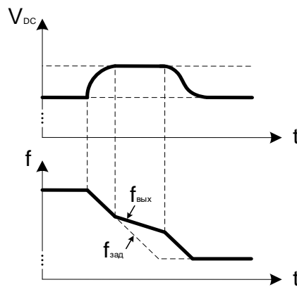
Рисунок 9-45 Ограничение перенапряжения звена DC
