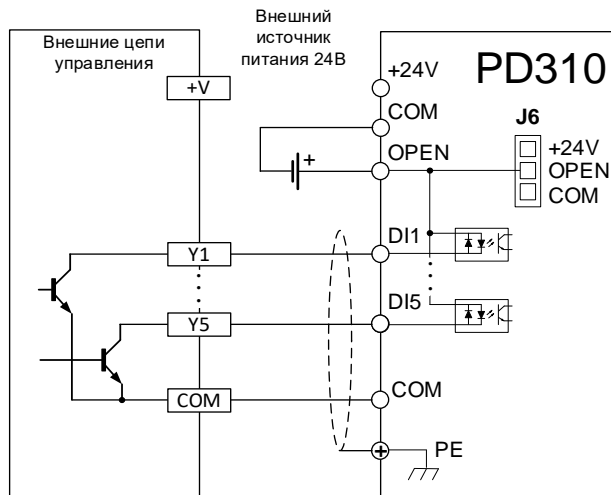
Рисунок 4-28 Режим NPN, использование внешнего источника питания
