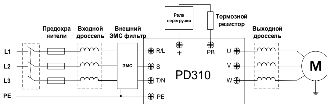
Рисунок 4-16 Схема подключения трехфазных моделей A2/A4/A7/D4
