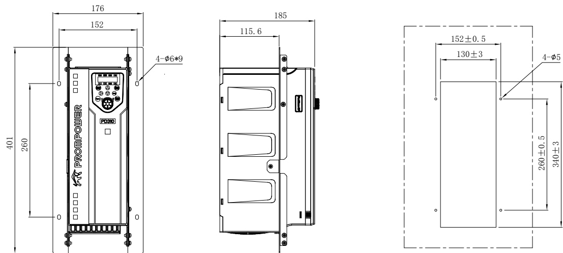
Рисунок 3-8 Монтажные размеры для установки в проем монтажной панели моделей 11 кВт
