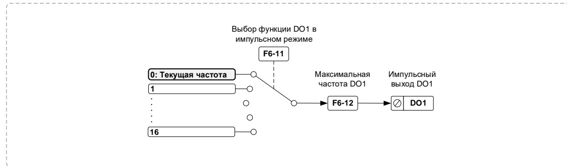
Работа DO1 в режиме импульсной последовательности (F6-05 = 0)
