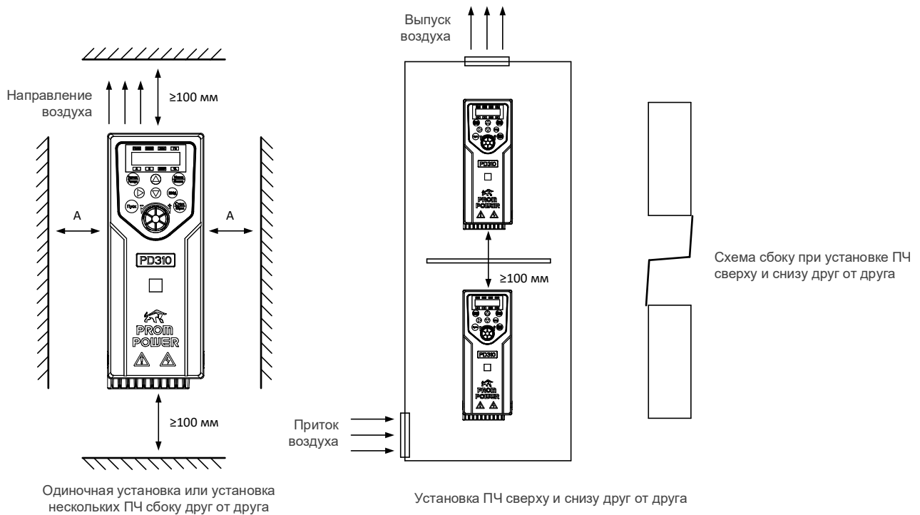
Рисунок 3-15 Установка преобразователя частоты
