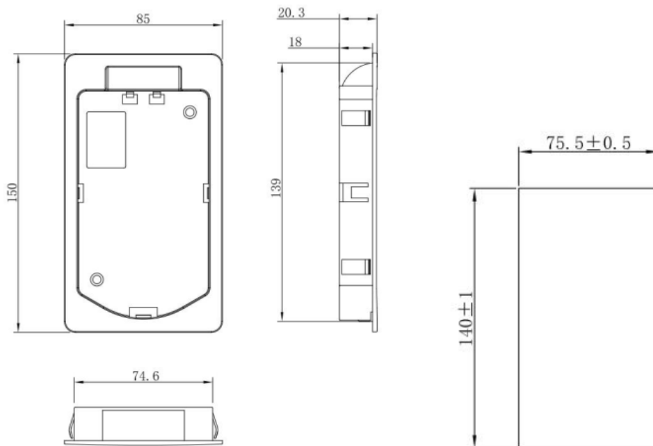
Рисунок 3-14 Габаритные размеры держателя кнопочной панели Keyboard bracket
