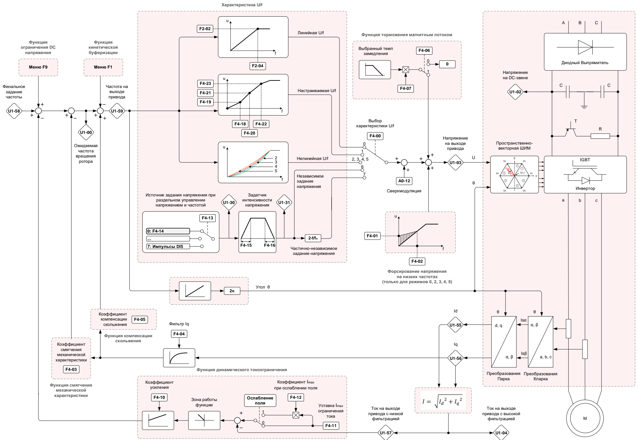
Рисунок 9-13 Структурная схема скалярной системы управления
