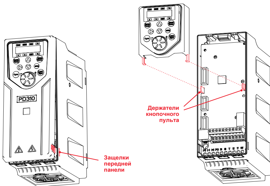
Рисунок 4-18 Снятие передней крышки и кнопочного пульта для моделей с пластиковым корпусом
