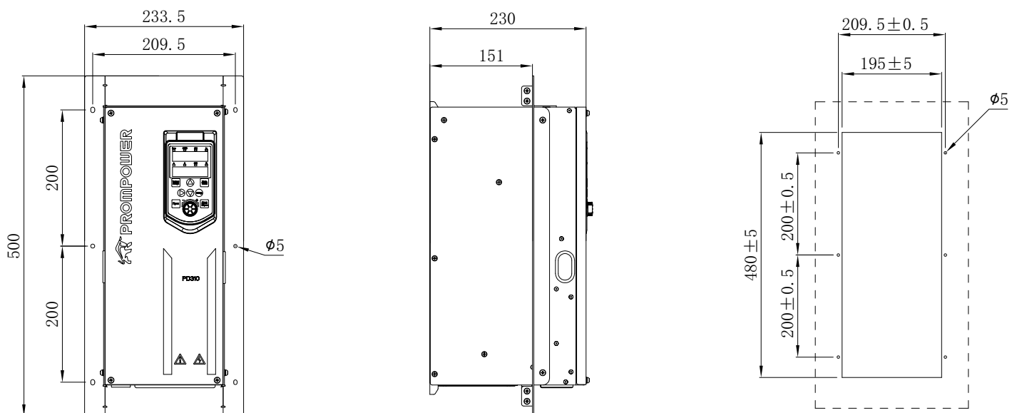
Рисунок 3-10 Монтажные размеры для установки в проем монтажной панели моделей 30-37 кВт
