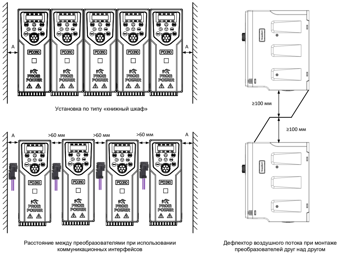
Рисунок 3-16 Установка преобразователя частоты
