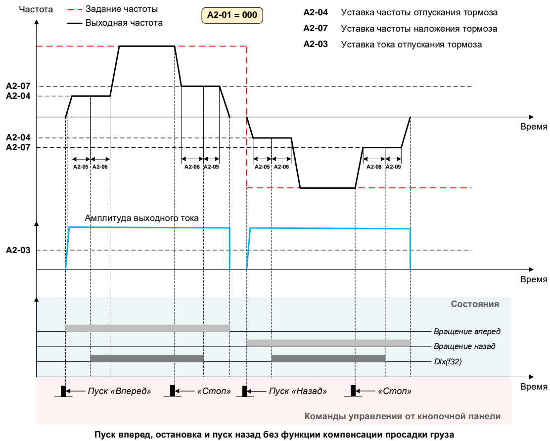
Рисунок 9-56 Временные диаграммы при использовании функции управления механическим тормозом без компенсации просадки груза и пропуска низких частот
