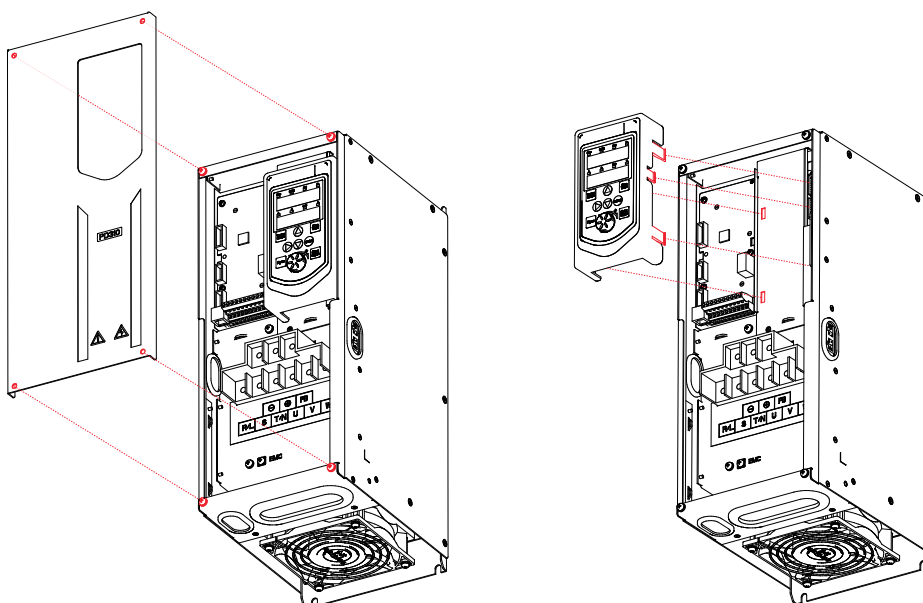
Рисунок 4-19 Снятие передней крышки и кнопочного пульта для моделей с металлическим корпусом
