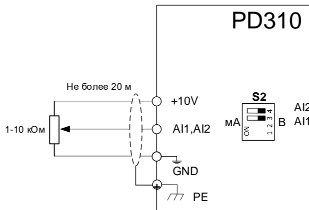
Рисунок 4-34 Схема подключения аналоговых сигналов в режиме 0~10 В
