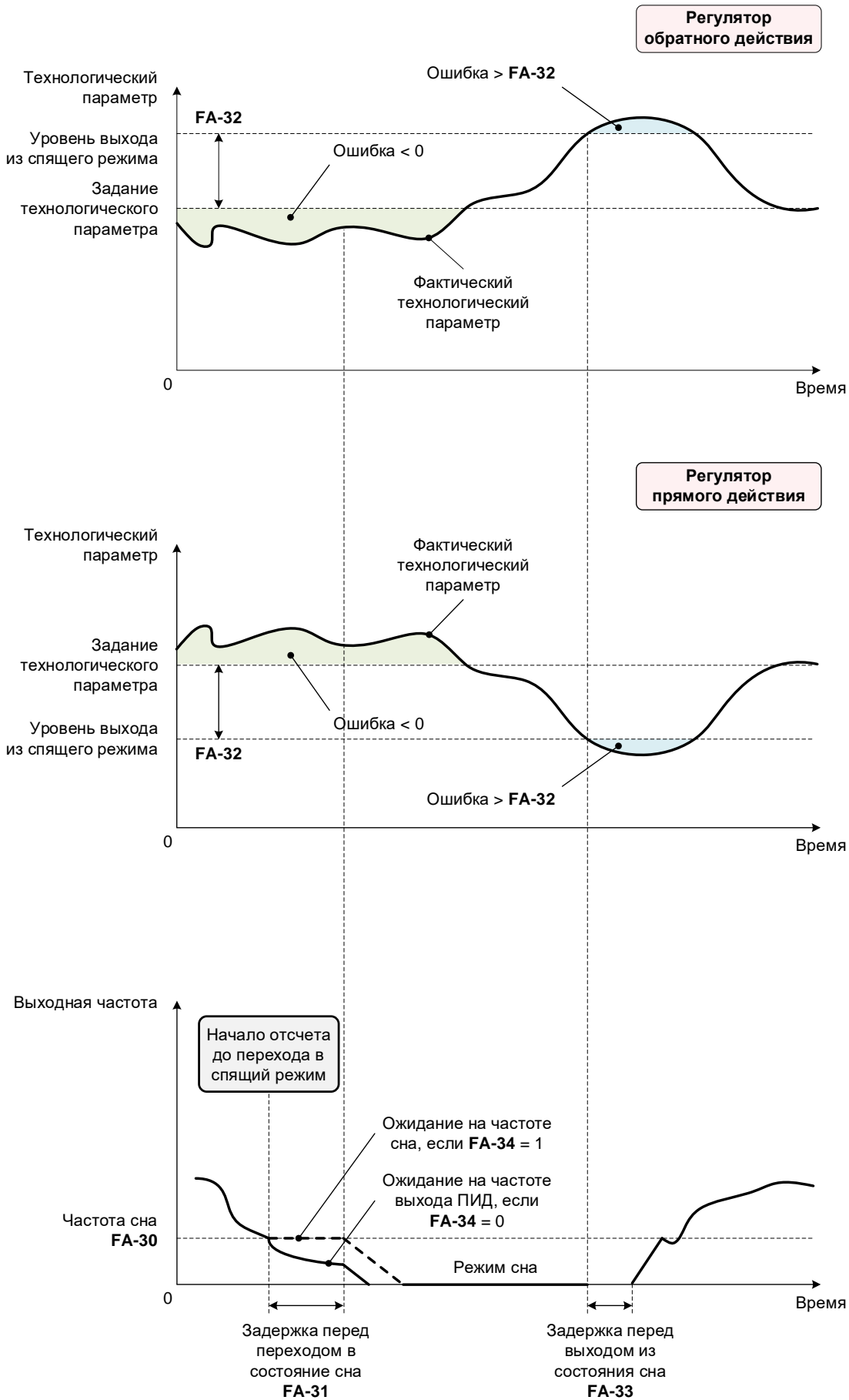
Рисунок 9-52 Временные диаграммы работы ПИД-регулятора прямого и обратного действия при входе в режим сна и выходе из него при FA-29 = 2
