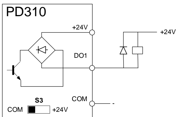
Рисунок 4-33 Схема подключения дискретного выхода с использованием внешнего источника питания в режиме NPN
