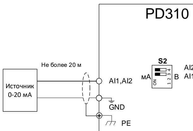
Рисунок 4-35 Схема подключения аналоговых сигналов в режиме 0~20 мА
