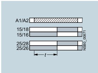
A с задержкой на включение
