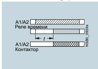
3RT1926-2C с задержкой на включение двужильное исполнение (варистор встроен)
