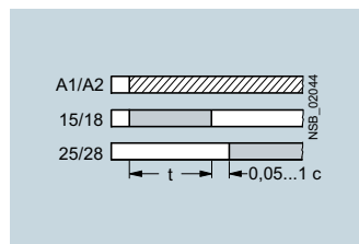
— 7PV1578 Функция «звезда-треугольник» 2)
