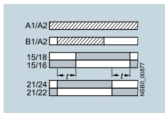
C•¹) 3RP2005-B с задержкой на включение и на выключение по управляющему сигналу и с мгновенным срабатыванием ( t = t_{an} = t_{ab} )
