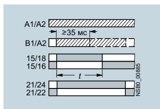
G•¹) 3RP2005-B с формированием импульсов по управляющему сигналу и с мгновенным срабатыванием (создание импульса на выходе независимо от продолжительности возбуждения)
