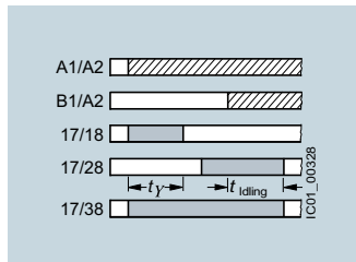
3RP2560-SW30, 3 НО, функция «звезда-треугольник» с функцией выгера (ldling)
