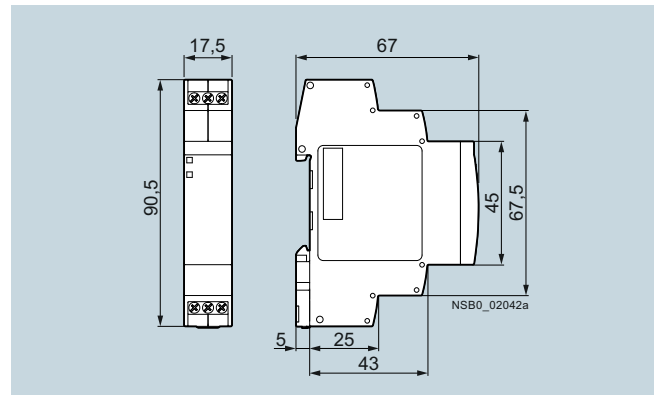
Размеры
