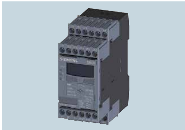
Цифровое реле контроля температуры SIRIUS 3RS1441 макс. для 3 датчиков
