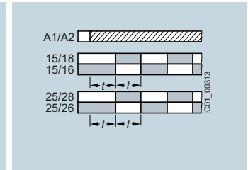
D формирование симметричного меандра (мигание, время "горения" равно времени "негорения"); начало с паузы ("негорения")
