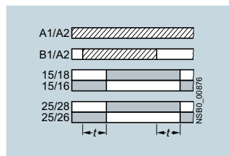
C¹) 3RP2005-B с задержкой на включение и на выключение по управляющему сигналу ( t = t_{an} = t_{ab} )
