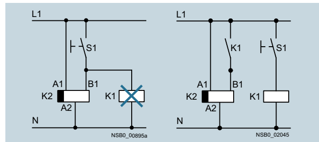
Схемы соединений
