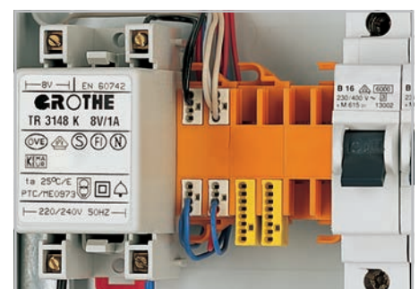
Монтаж на DIN-рейку 35 мм (дверной звонок)
