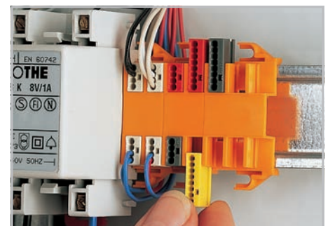
Вставка соединителя в монтажный адаптер.
