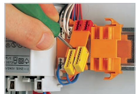
Извлечение монтажного адаптера из DIN-рейки.
